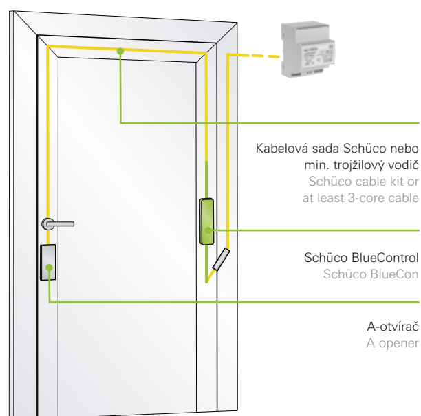
Příklad: instalace do dveřního křídla s A-otvíračem Example: Installation in the leaf frame with A opener
