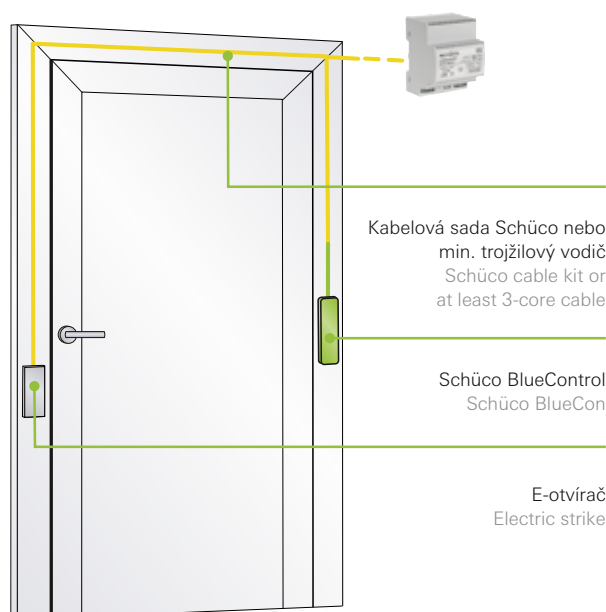
Příklad: instalace do dveřní zárubně s E-otvíračem Example: Installation in the outer frame with electric strike
